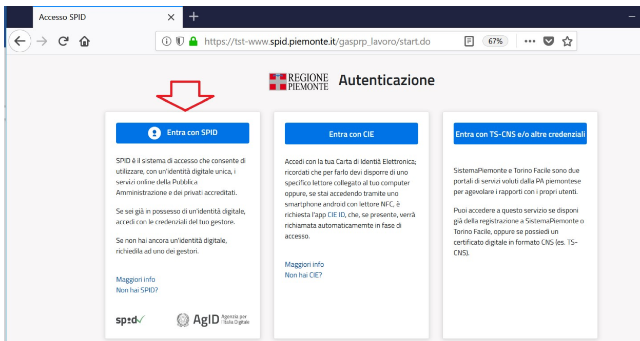
Figura 2 - Autenticazione
