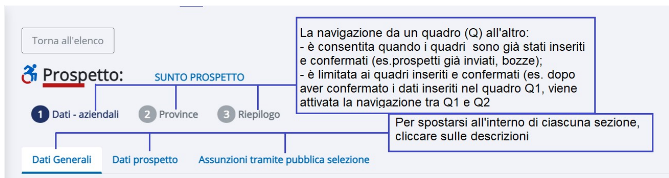
Figura 10 – Navigazione prospetto
