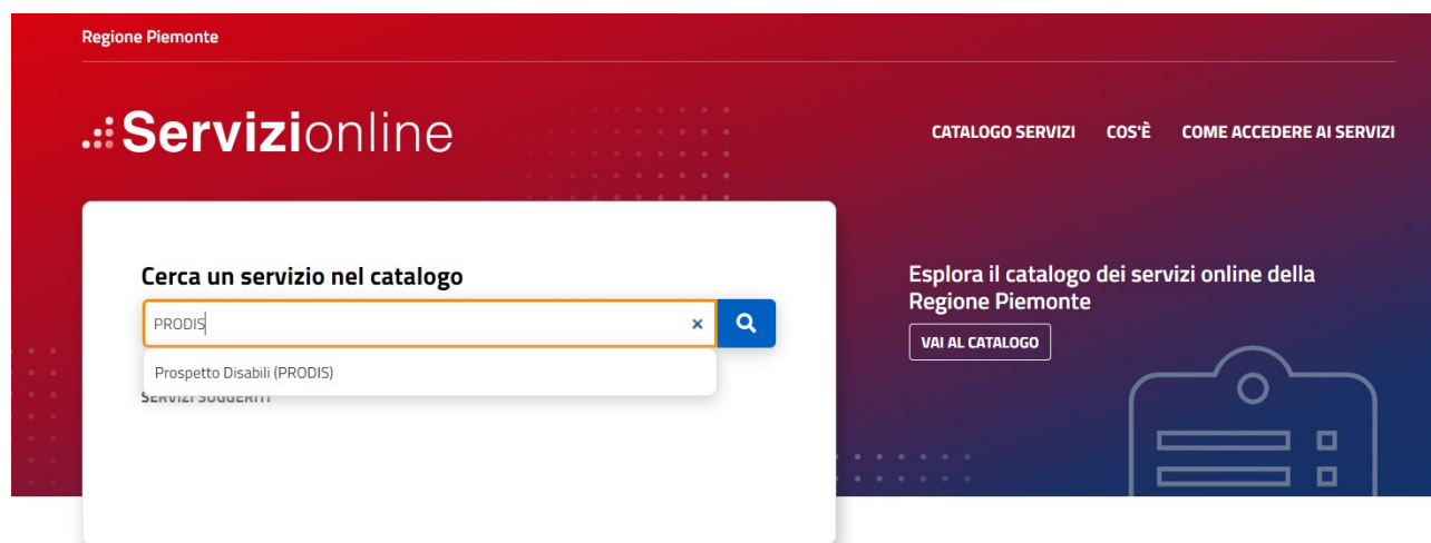
Figura 2 – Servizi online
