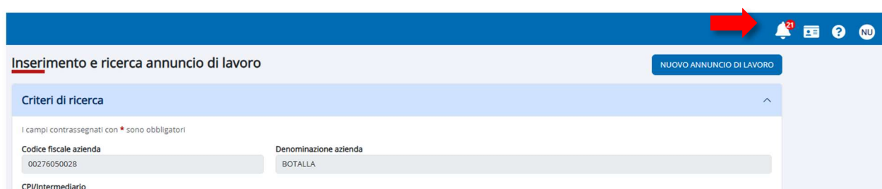
Figura 48 – Notifiche
