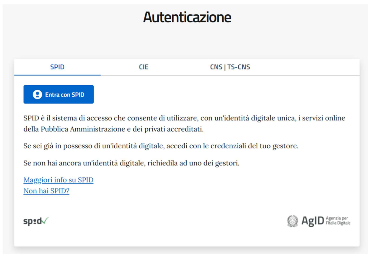
Figura 3 – Autenticazione
