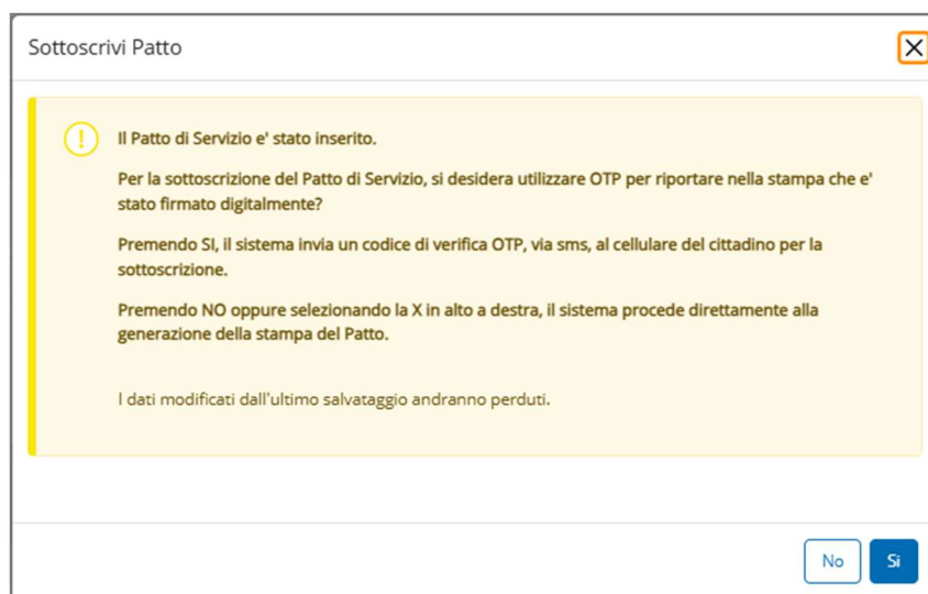
Figura 28 – Sottoscrivi Patto
