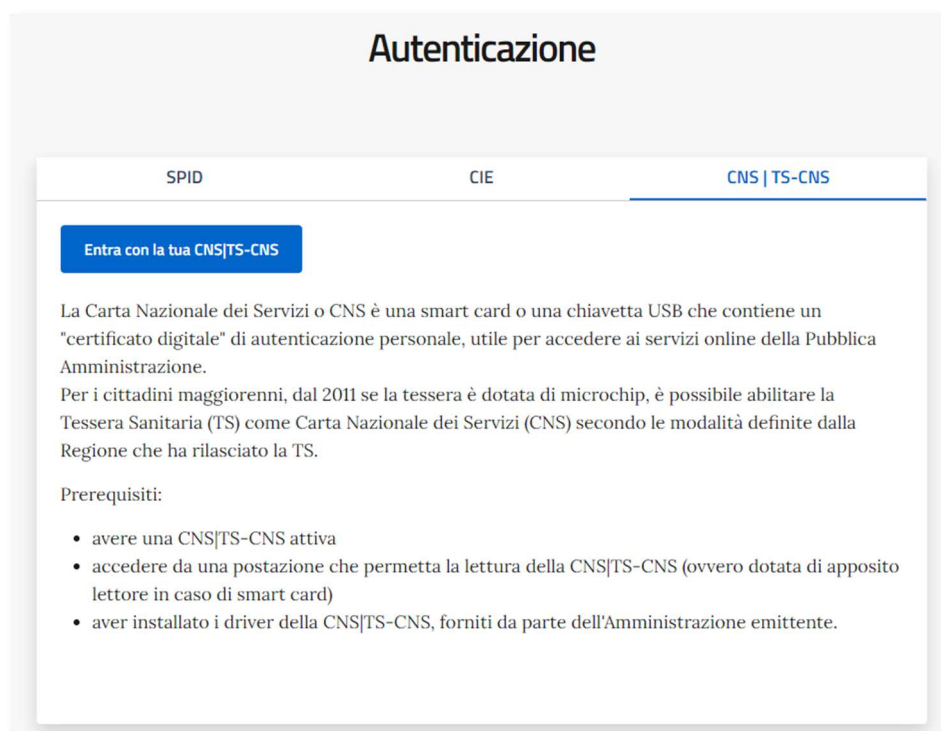
Figura 2 - Autenticazione
